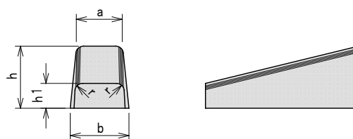
両面歩車道境界ブロック (斜1段落し)
