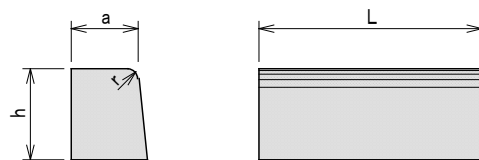
歩車道境界ブロック
