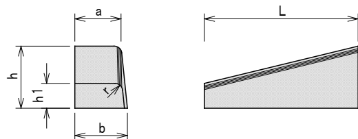
歩車道境界ブロック (斜1段落し)
