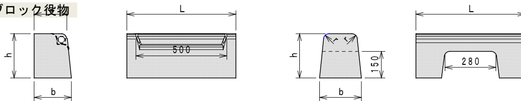
歩車道境界ブロック (斜1段落し)
