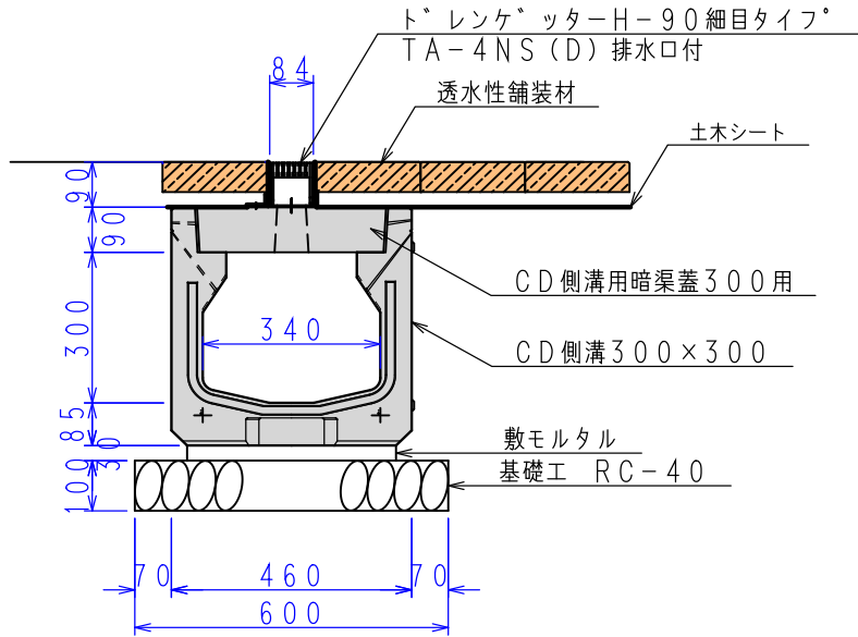
標準断面図
